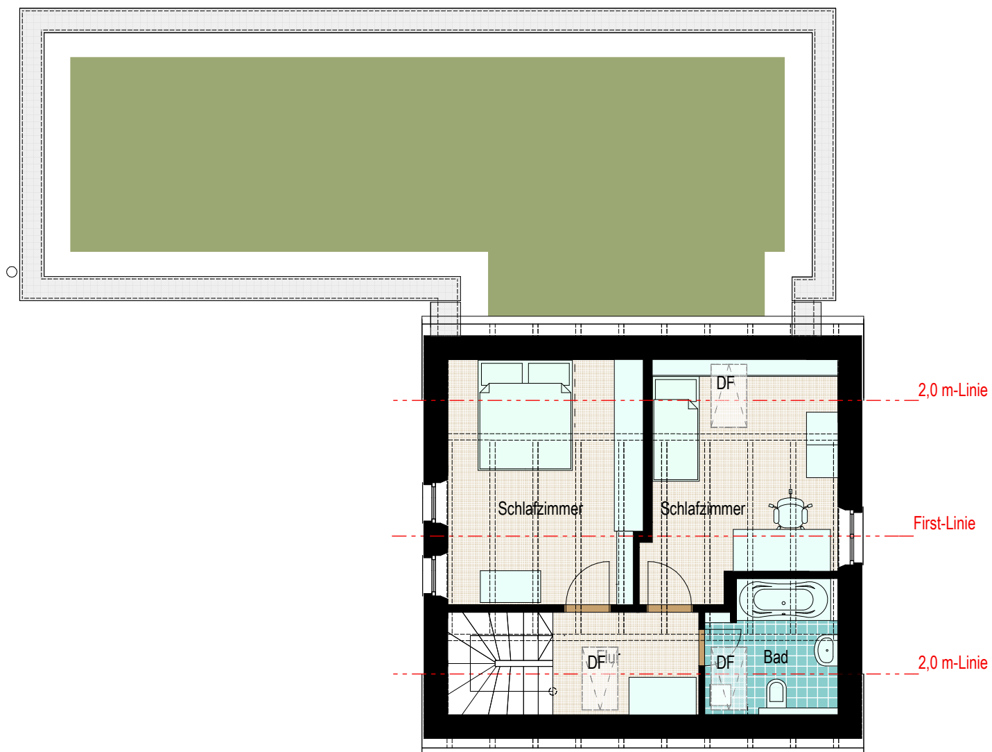
Dachgeschoss
