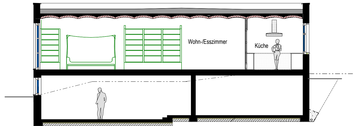
Längsschnitt
