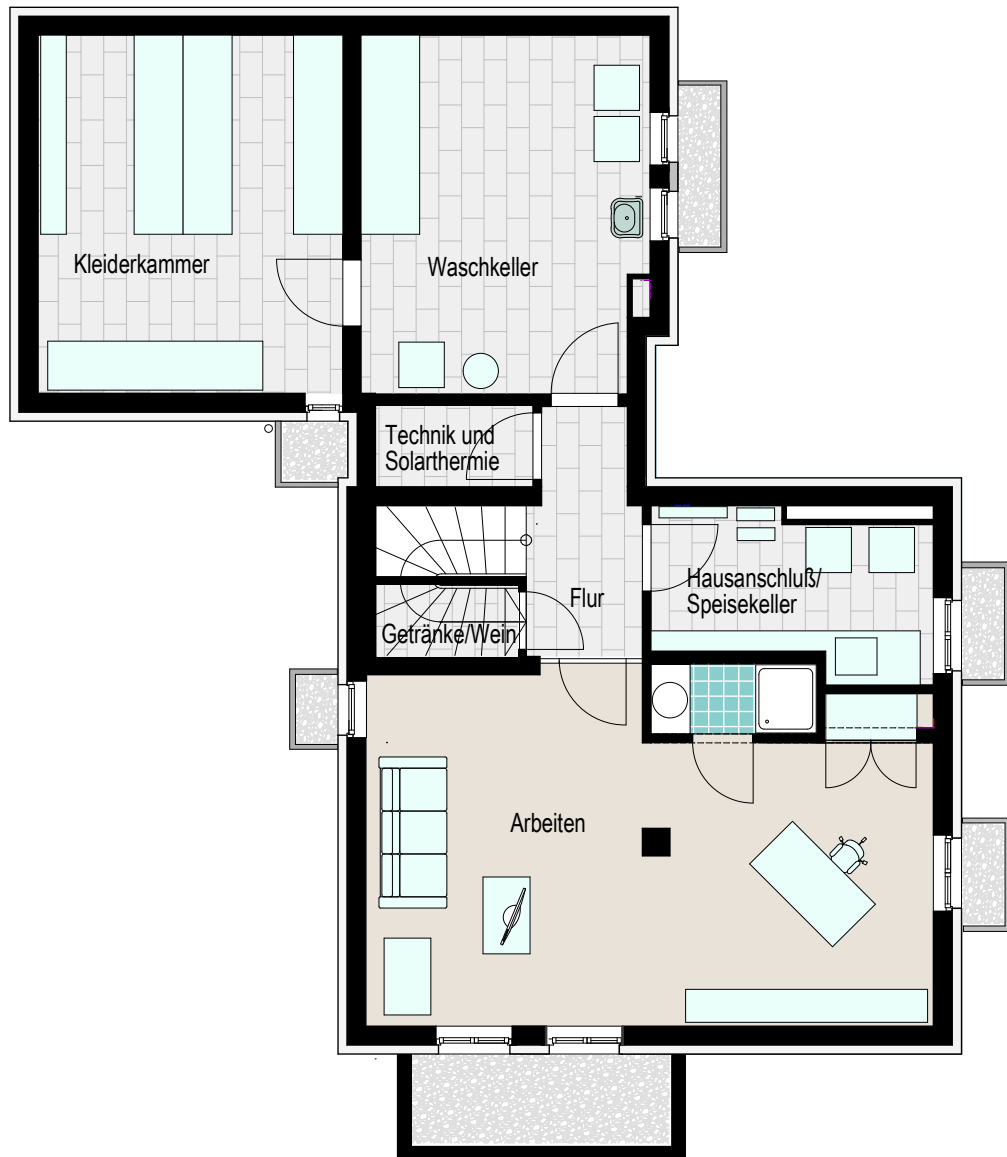
Kellergeschoss
