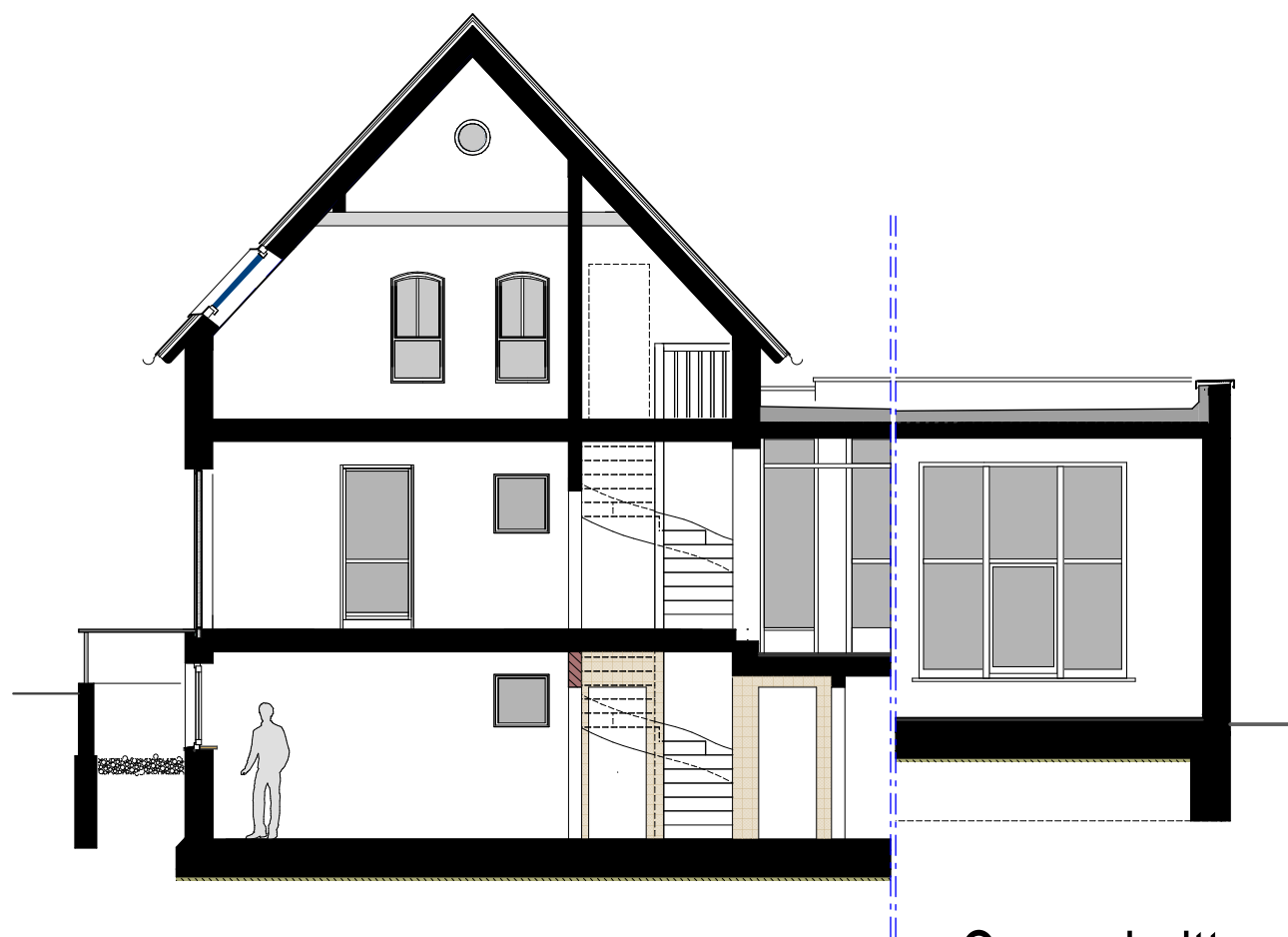
Querschnitt
