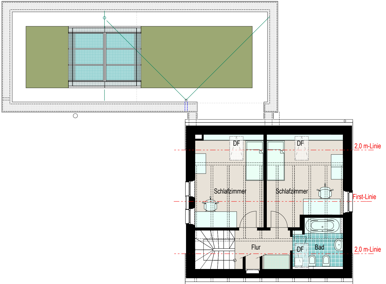
Dachgeschoss
