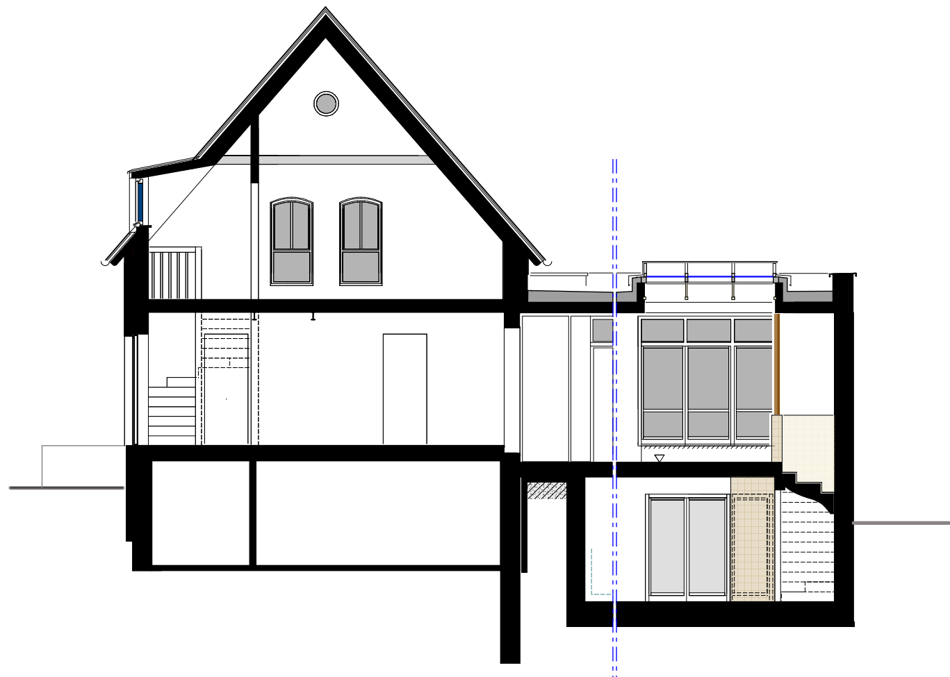
Querschnitt
